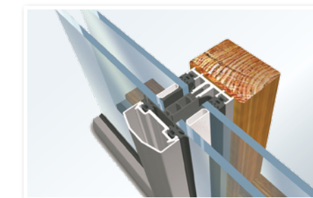
ALUMERO AT 500 F mit Aufsatzpfosten aus Holz
